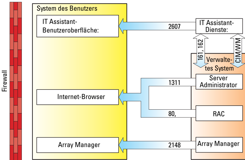
Abbildung 11-1. Typische Installation hinter einer Firewall
