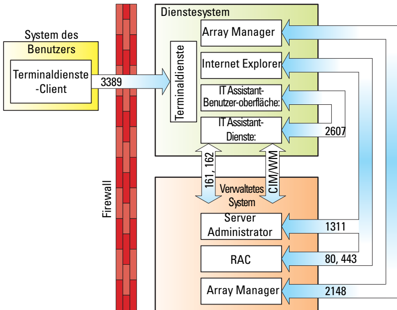
Abbildung 11-2. Terminaldienste für zusätzliche Sicherheit verwenden
